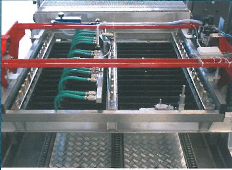
Testa di presa Pick-up head Cabezal de toma
